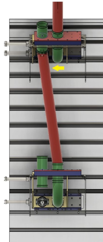
2、中段打設の準備 打設管を左へスライド
