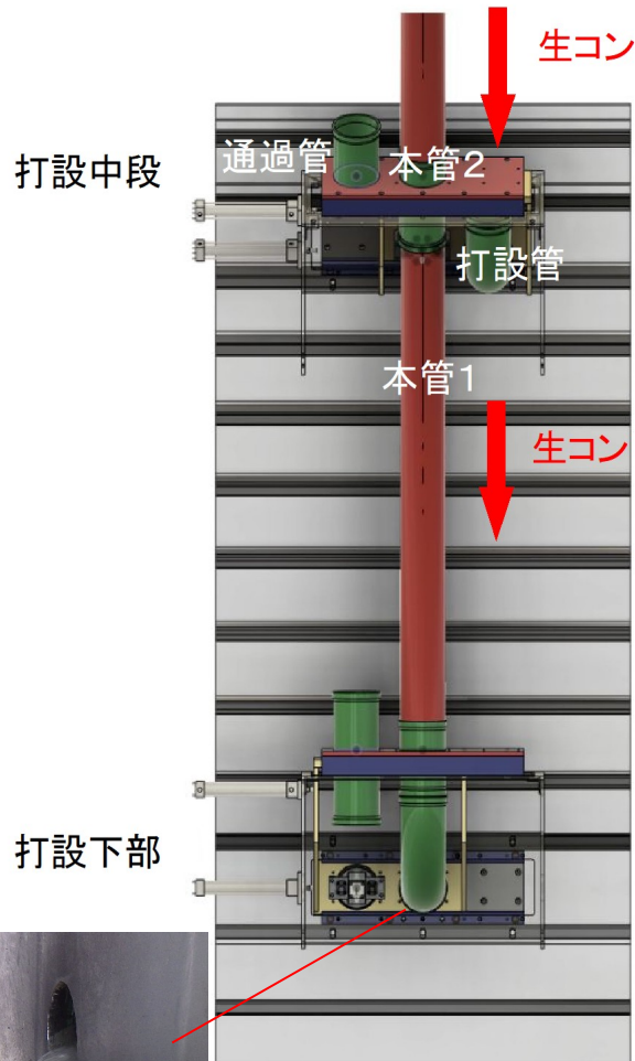
1、下部打設 生コンは本管2⇒本管1⇒打設口
